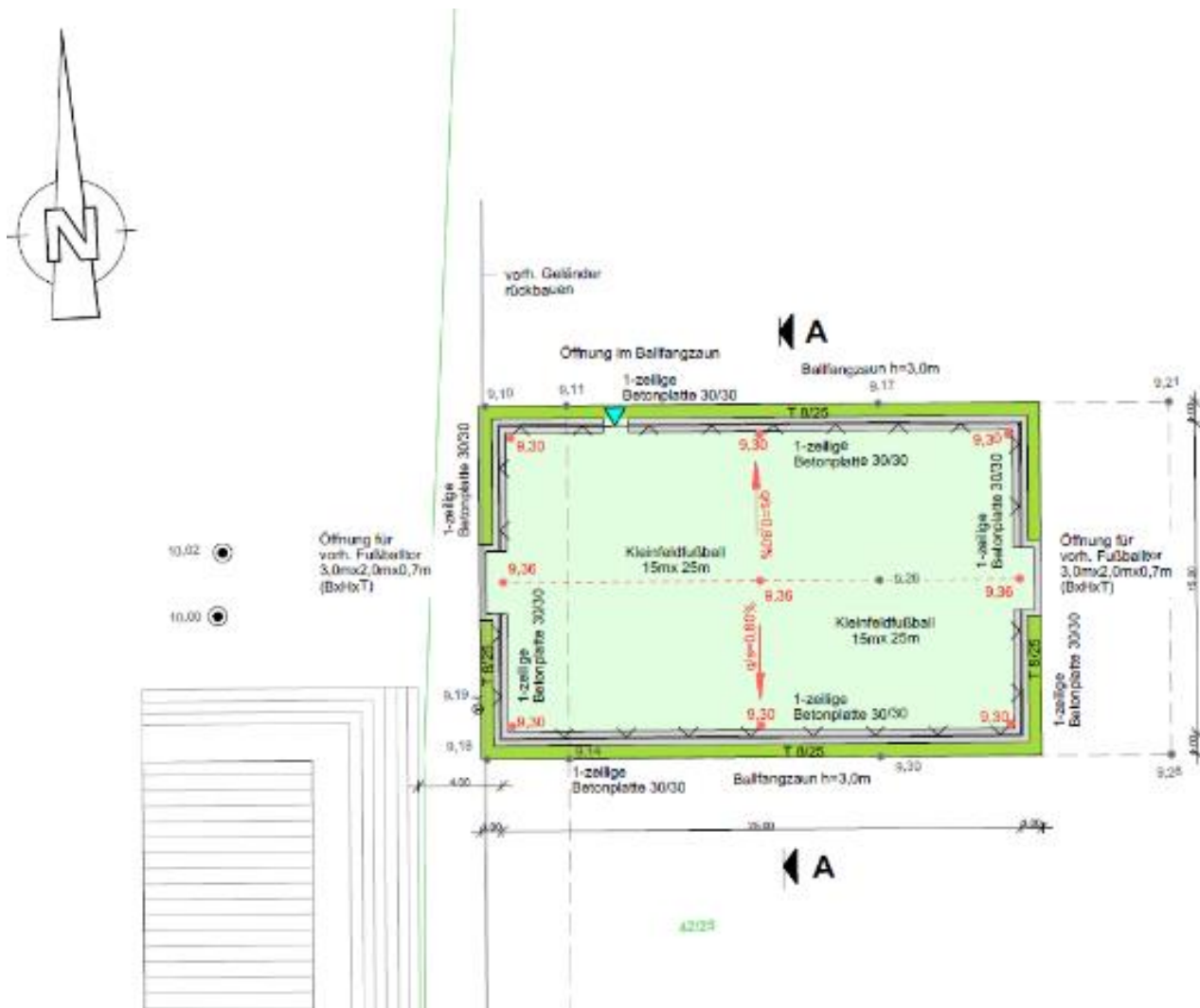
Foto 2: Lageplan
