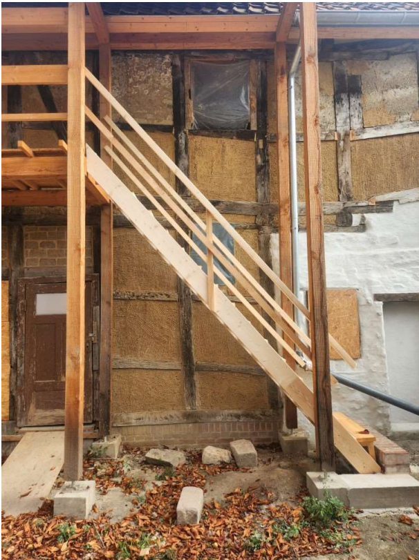
Vorübergehend installierte Bautreppe für ein besseres Handling der folgenden Gewerke
